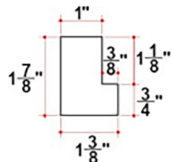
Zen L (ZL)
