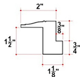
Deco Trim / K35
