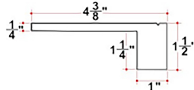
Small Zen Sill Cap (SZSC)
