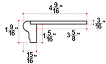
AJ 520 Sill Cap
