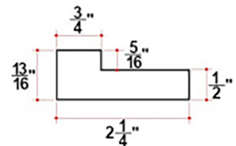
Zen Sill Piece (ZSP)
