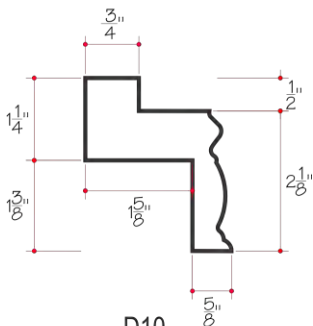
D10 Z-FRAME
