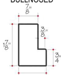
L14 L-FRAME
