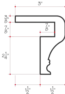
SILL CAP
