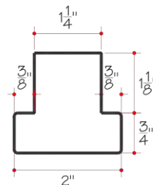
L16 T-POST
