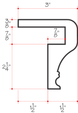
SILL CAP
