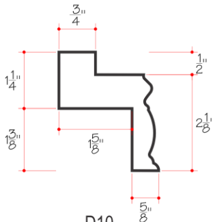
D10 Z-FRAME
