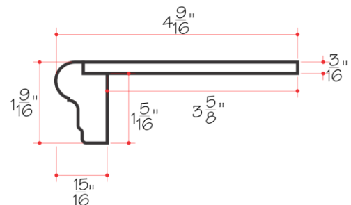
SILL CAP
